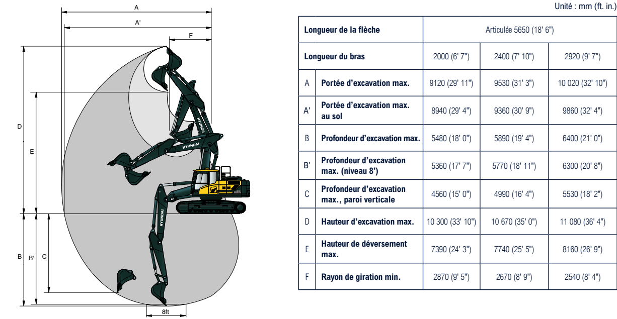
Plage de travail de la pelle articulée (niveau 8")
